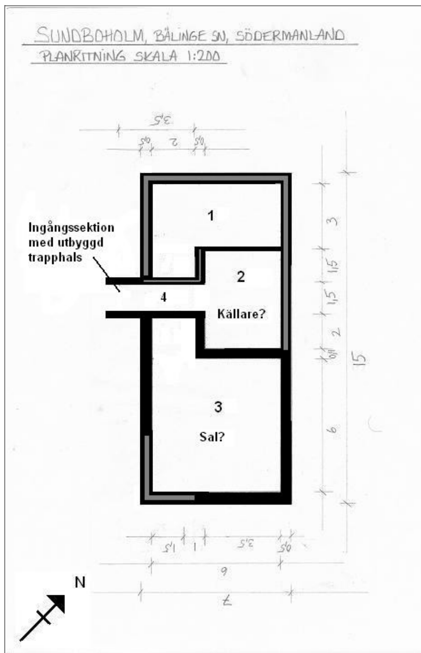
Illustration 1: Fig. 2: Planritning av Sundboholm, Bälinge sn i skala 1:200. Ritningen är sammanställd efter fornminnesregistrets uppgifter (FMIS, Bälinge 60:1), Christian Lovéns planritning (Lovén 2000:50) och efter egna observationer vid besök av platsen. Den visar grunden och en tolkning av rummens funktion och indelning. Grått streckade partier är osäkra. Skiss av förf.
